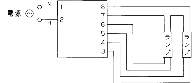
結線図
