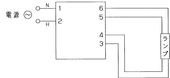
結線図
