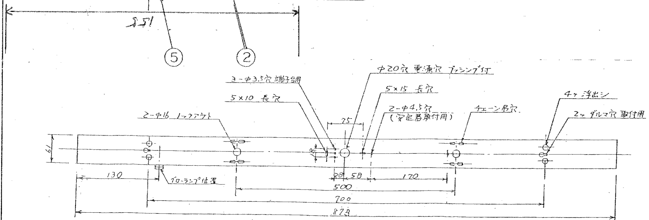
取付背面図 S=1/5
