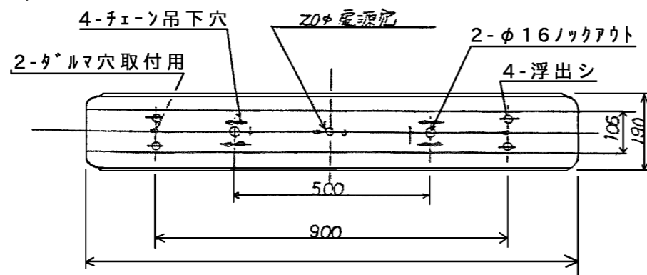
取付背面図 S=1/10
