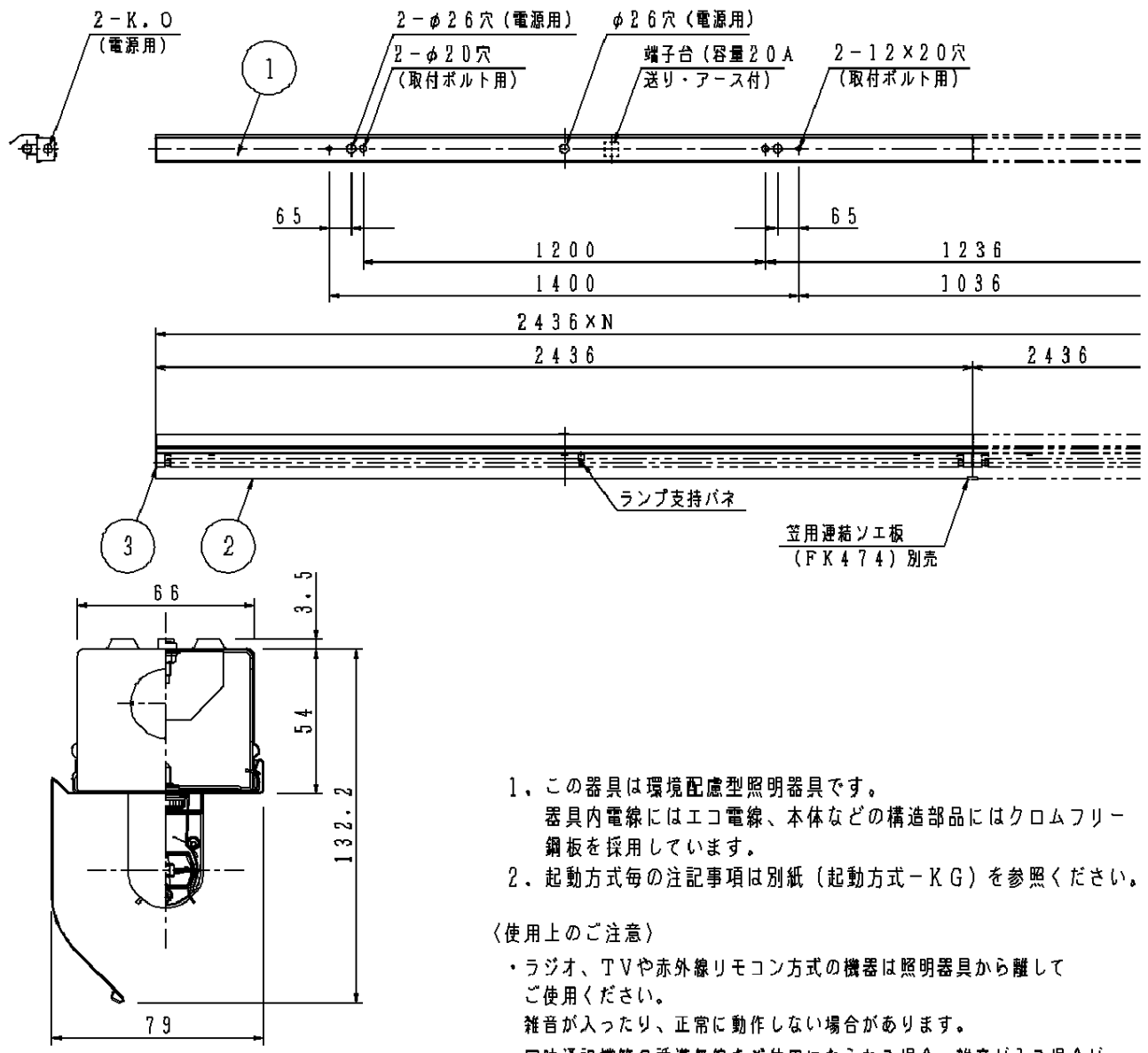
断面詳細図
