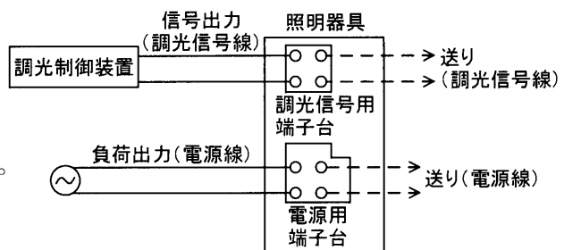
調光制御装置との結線図
