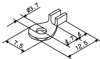
連続端子 (日本圧着端子製SRA-50T-3.7)
