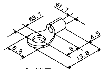
バラ端子 (ニチフ製1.25-3.5 M)
