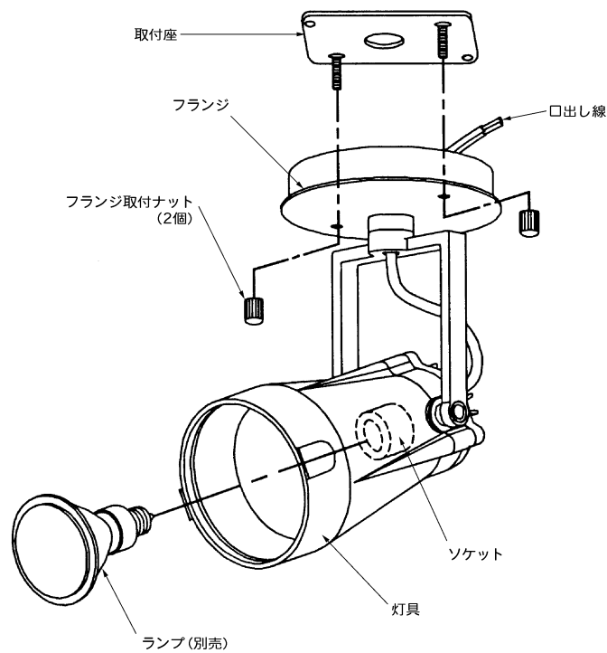
上図は器具の一部を簡略化しています。
