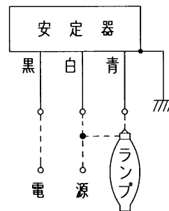
結線図
