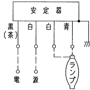
結線図
