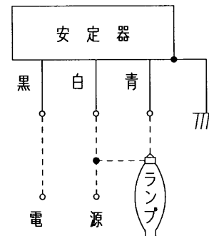
結線図
