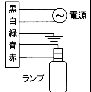
結線図
