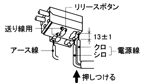
(適合電線φ1.6,φ2.0単線) 第2図
