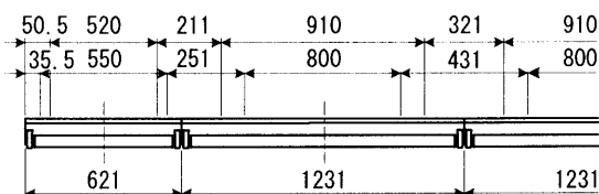
連結寸法図
