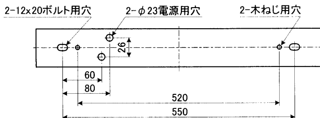
背面仕様図
