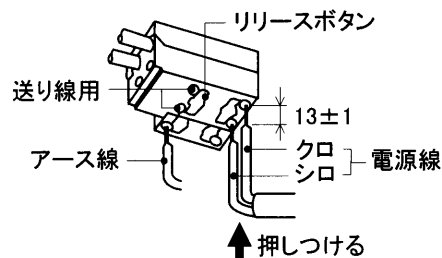
(適合電線φ1.6, φ2.0 単線) 第1図
