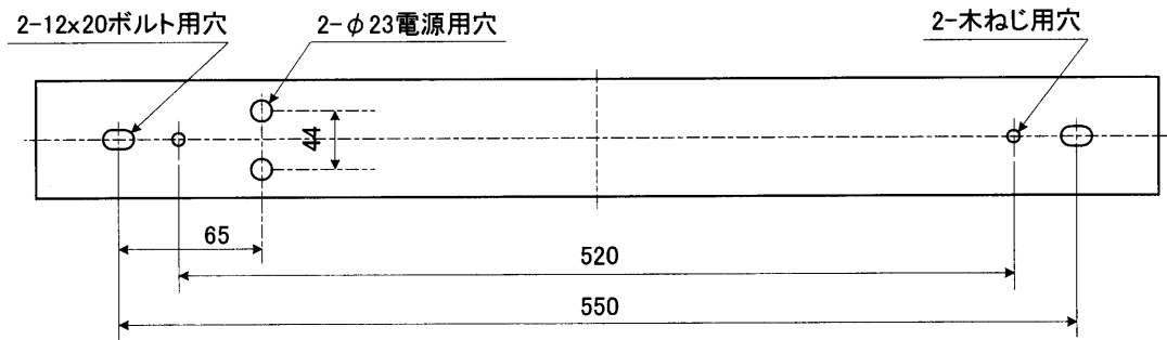
背面仕様図
