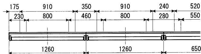
連結寸法図
