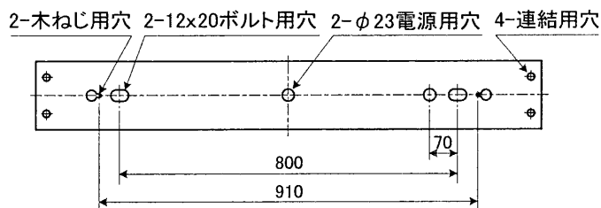
背面仕様図
