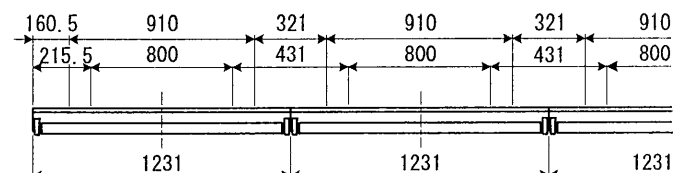
連結寸法図
