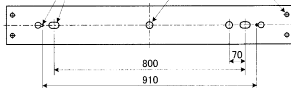
背面仕様図
