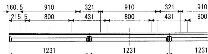
連結寸法図
