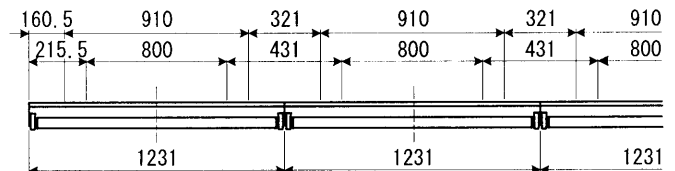
背面仕様図
