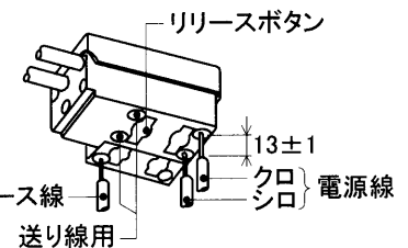
(適合電線φ1.6,φ2.0単線) 第4図
