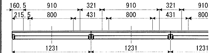
連結寸法図
