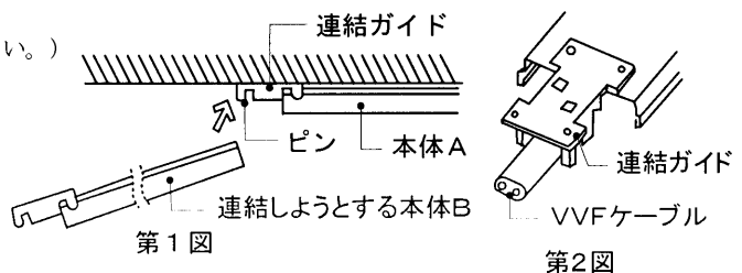
連結寸法図
