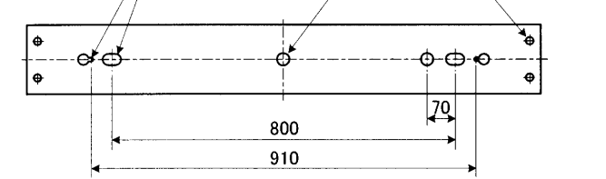
背面仕様図
