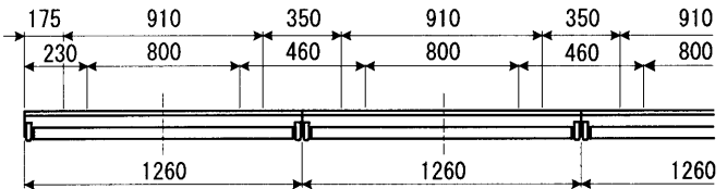
連結寸法図
