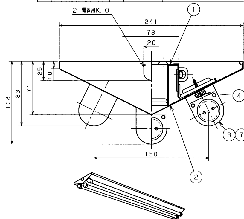
連結ガイド付
