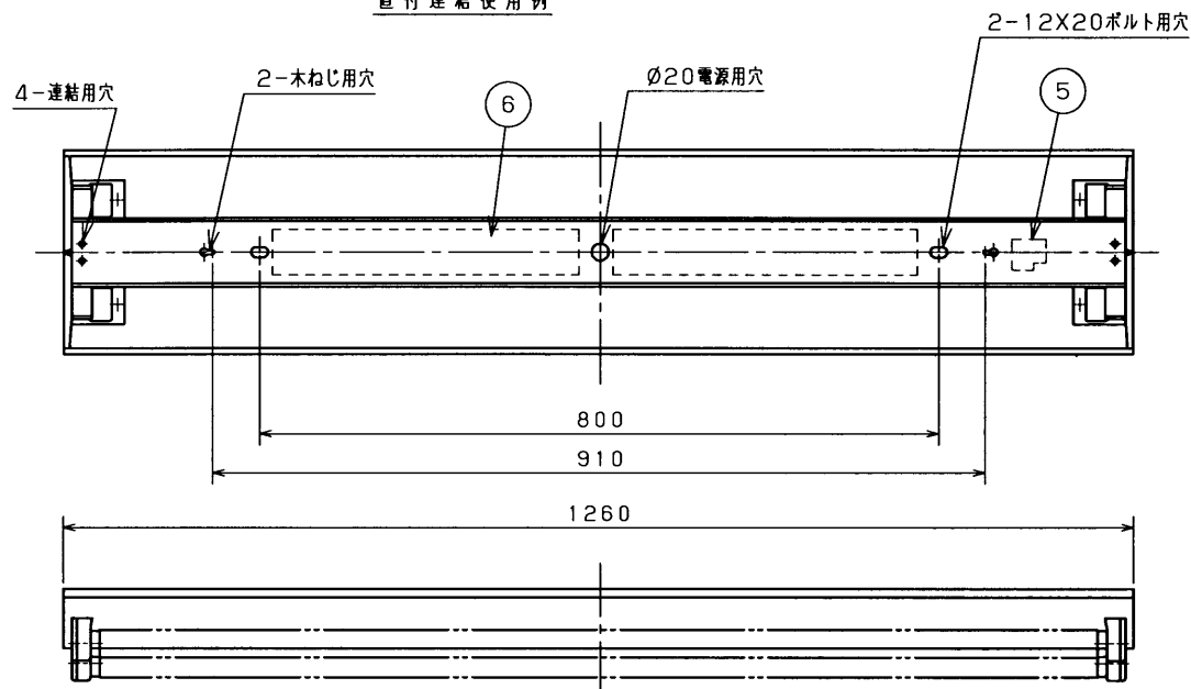
直付連結使用例
