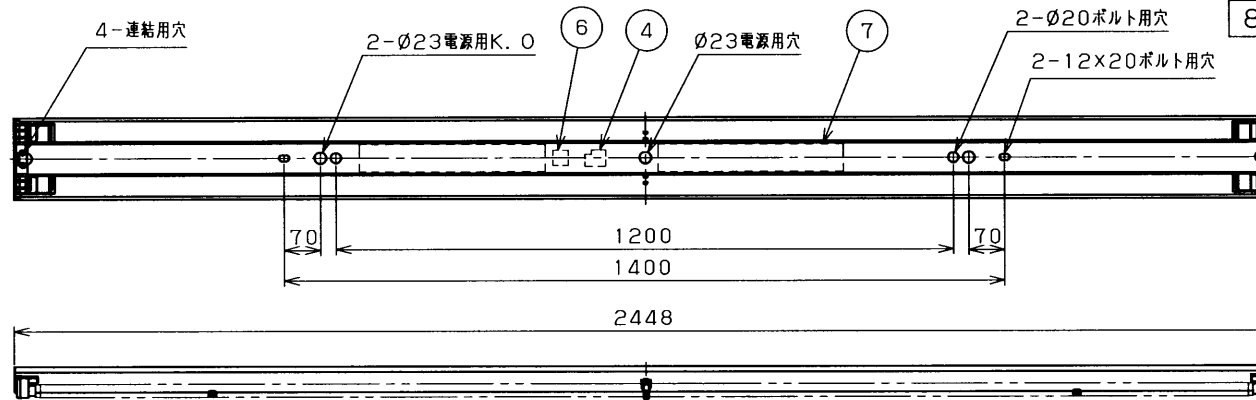
直付連結使用例
