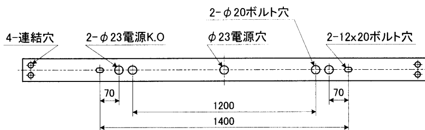
背面仕様図
