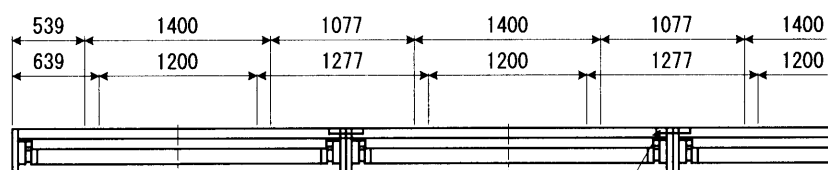
連結寸法図
