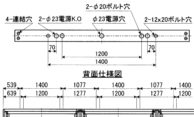
連結寸法図
