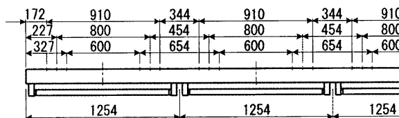
連結寸法図
