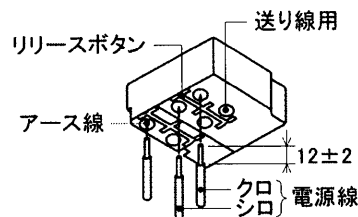
(適合電線φ1.6, φ2.0単線) 第4図
