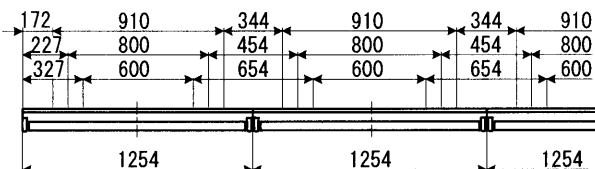
連結寸法図
