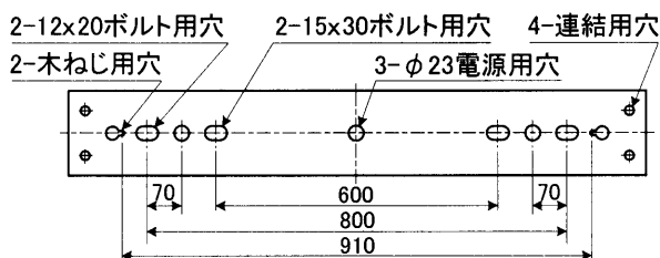
背面仕様図
