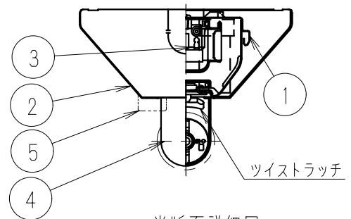
半断面詳細図
