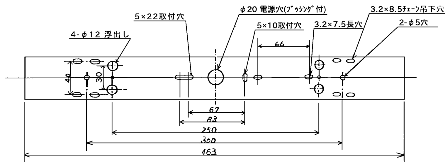
取付背面図 S=1/2
