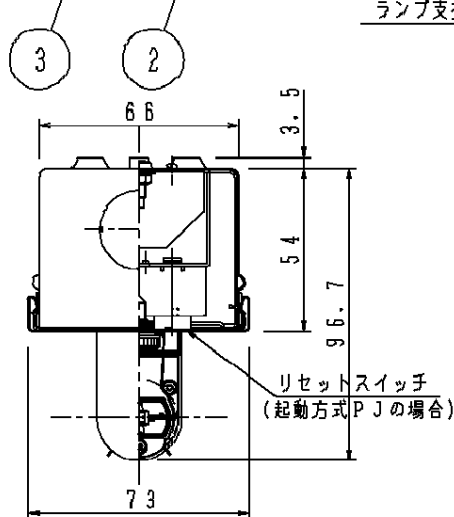
断面詳細図
