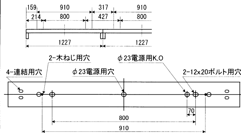
背面仕様図
