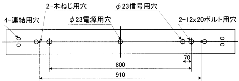
背面仕様図
