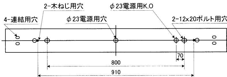
背面仕様図
