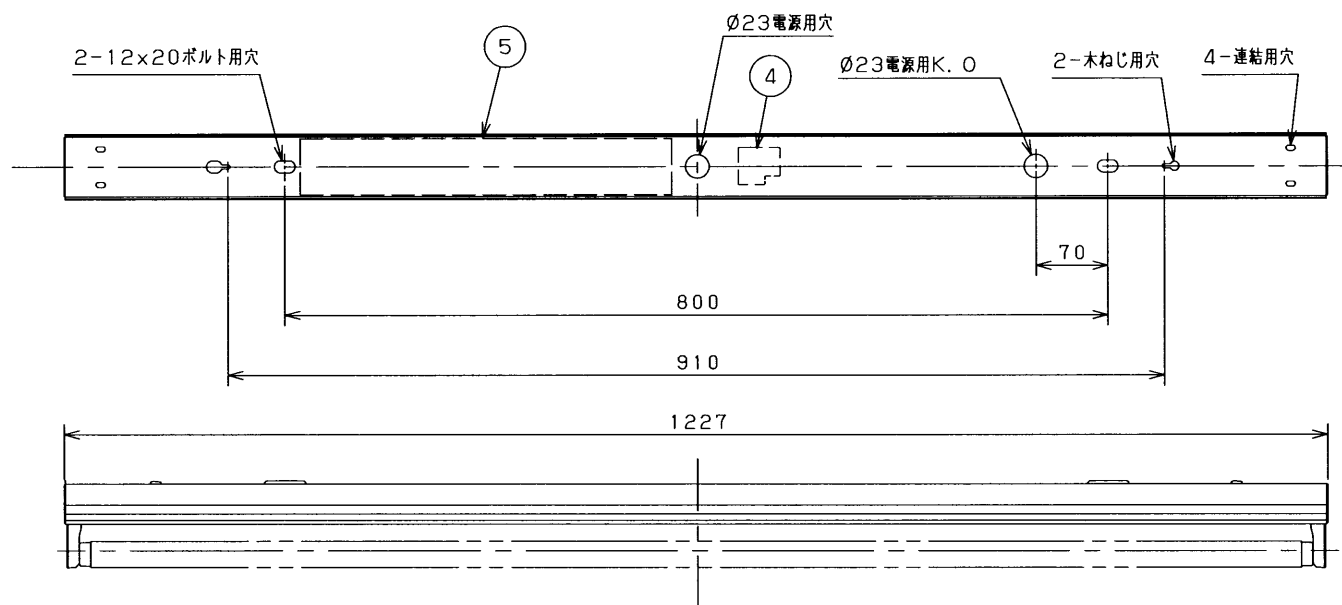
取付ボルトの器具内寸法
