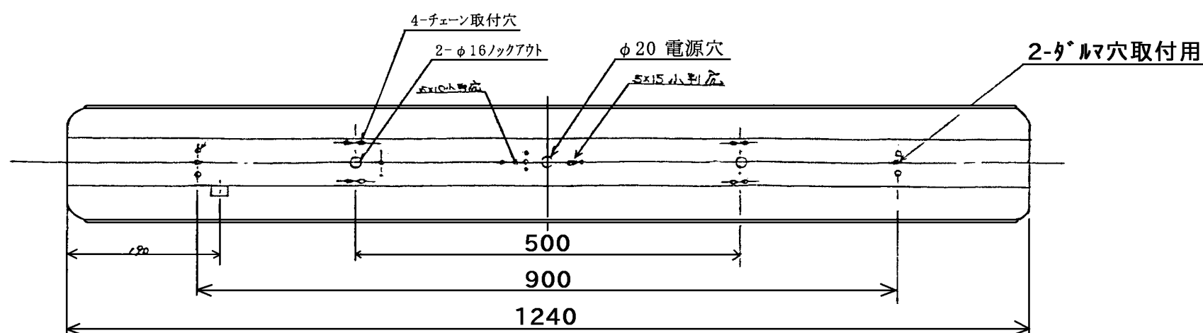
取付背面図 S=1/5
