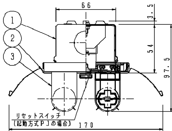
断面詳細図
