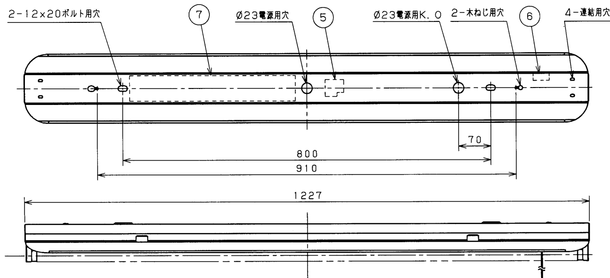
取付けボルトの器具内寸法
