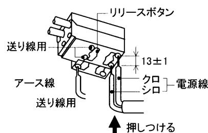
(適合電線φ1.6, φ2.0 単線) 第3図
