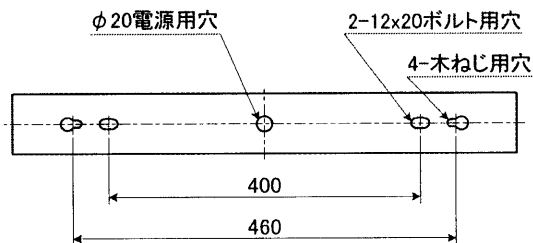
背面仕様図
