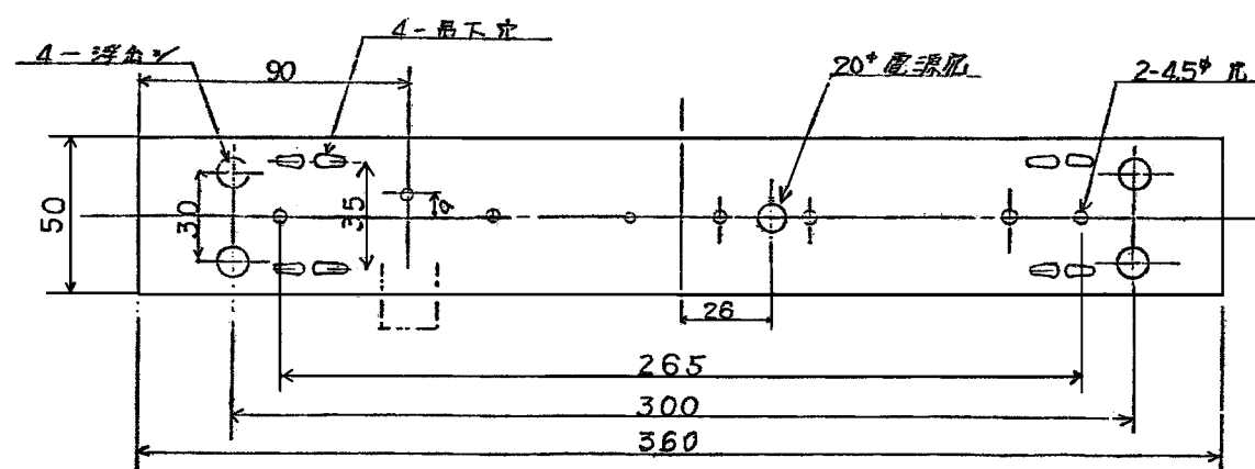
取付背図 s=1/2
