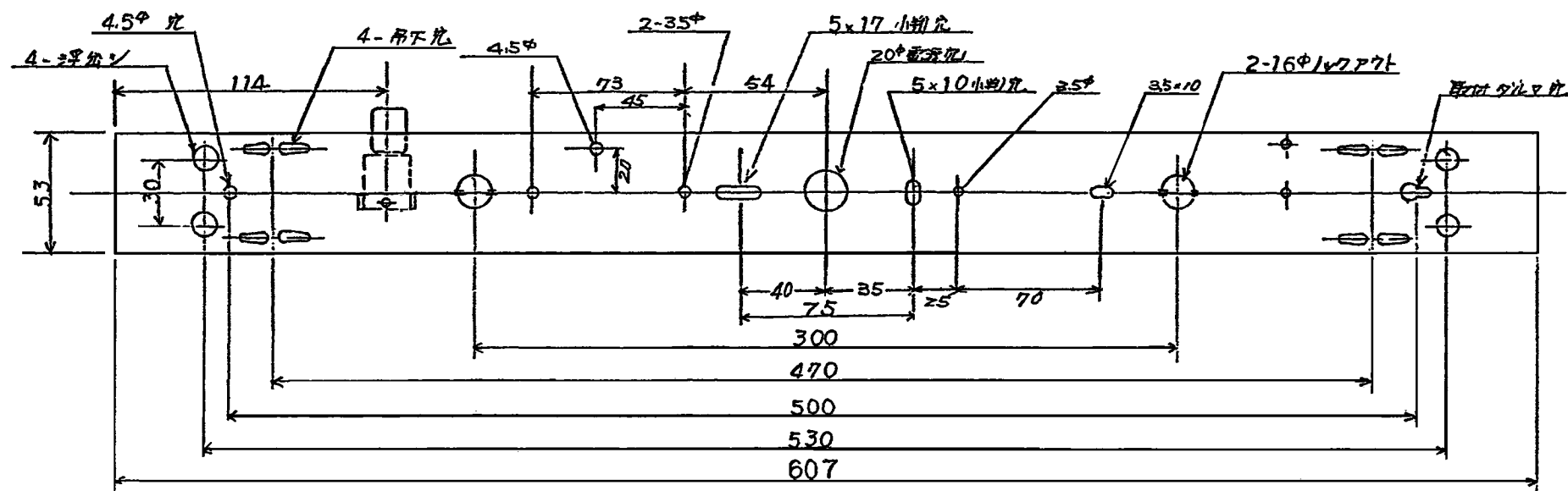
取付背面図5-1/2
