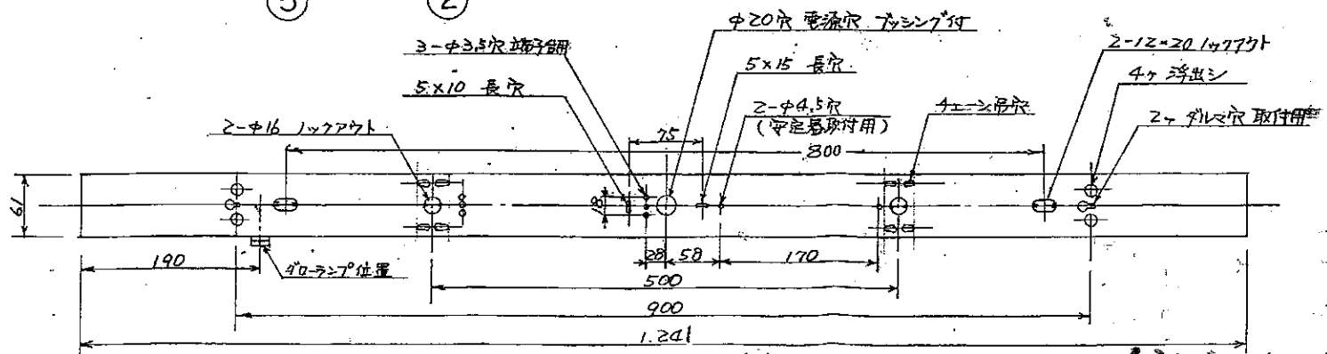
取付背面図 S=1/5
