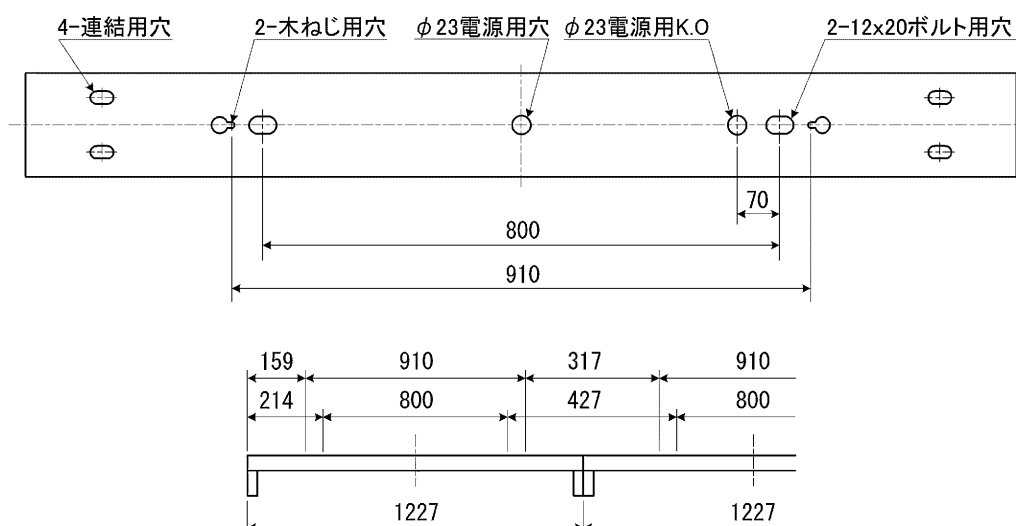
直付連結使用例
