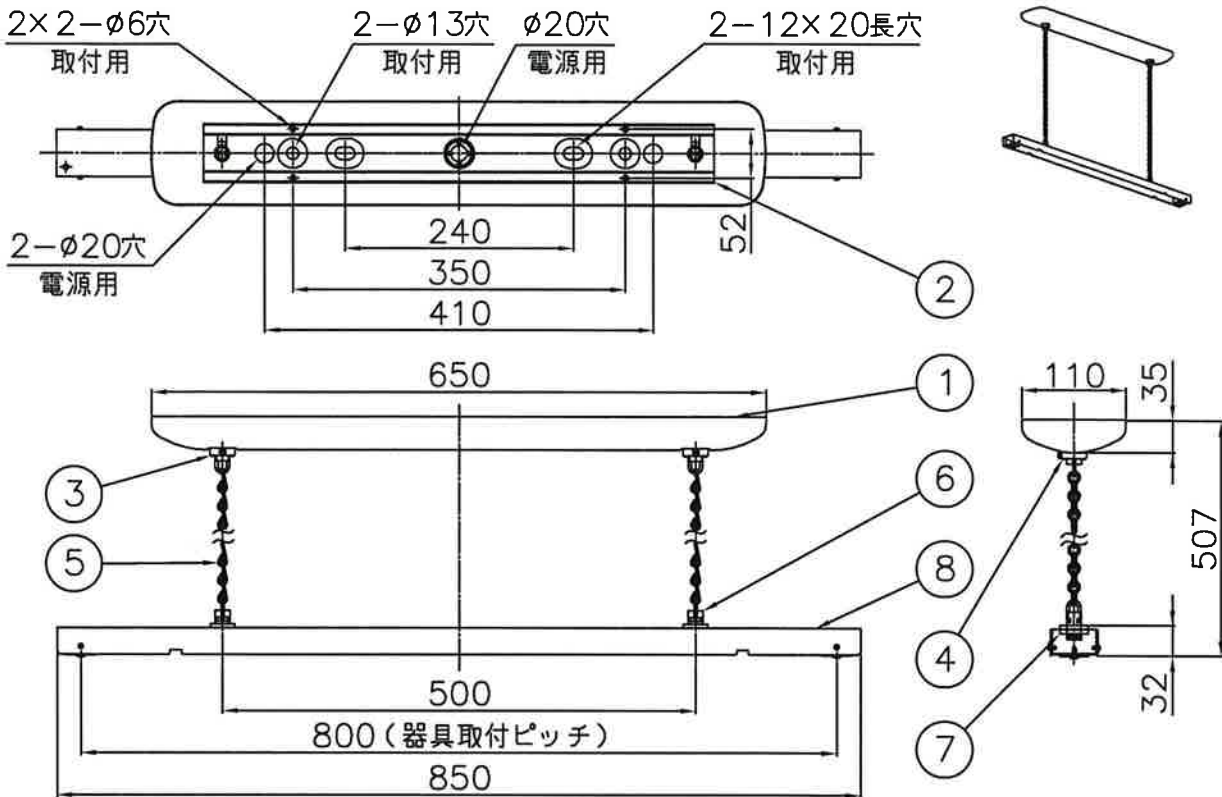
断面詳細図1/3
