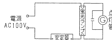
結線図
