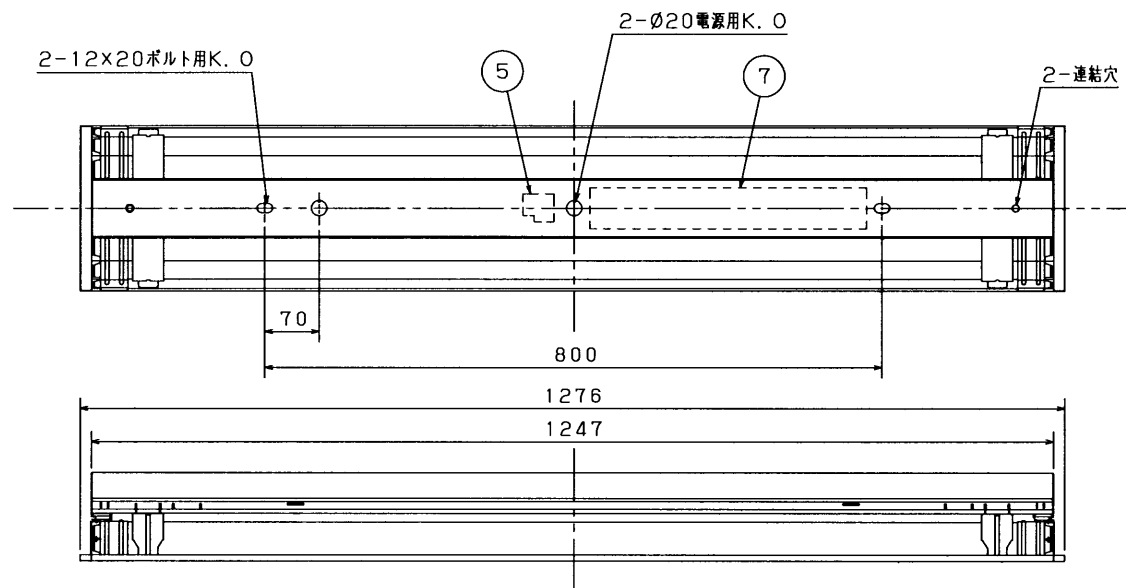
埋込穴寸法
