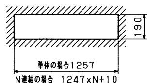
埋込寸法
