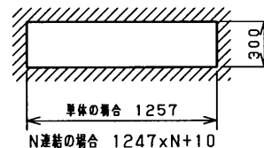
埋込穴寸法
