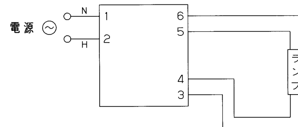
結線図
