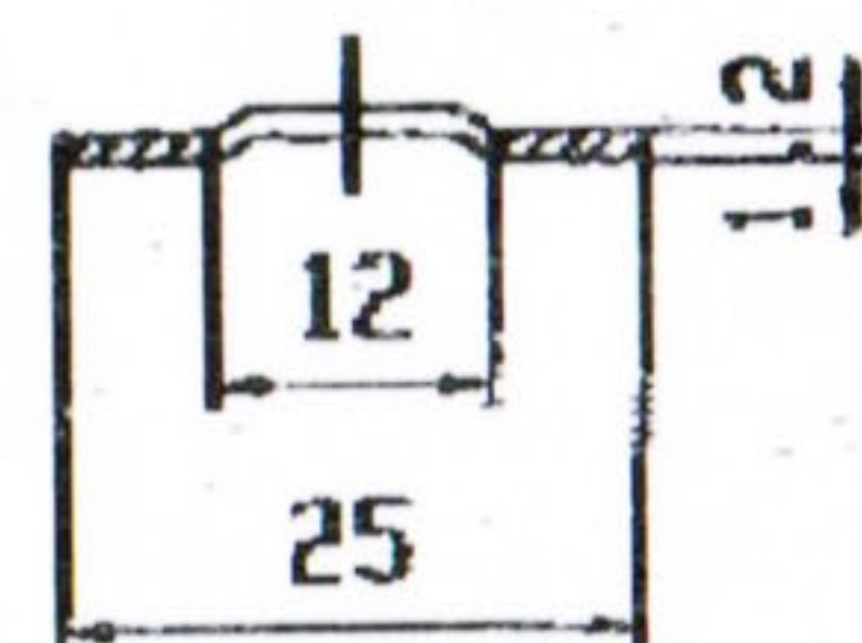
AA断面図
